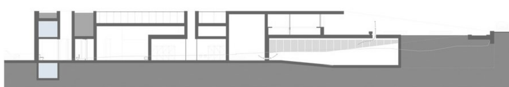
A-A CORTE LONGITUDINAL
