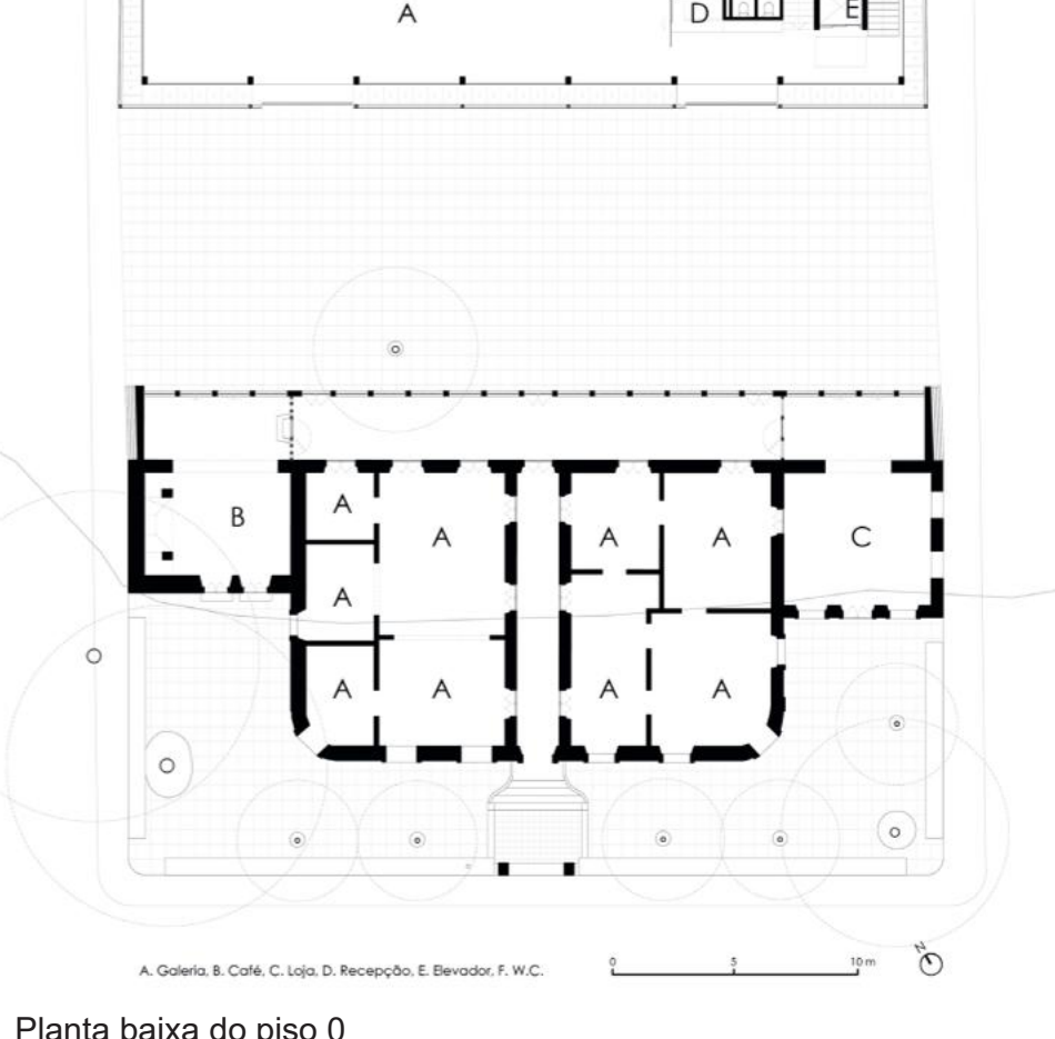
Planta baixa do piso 0
