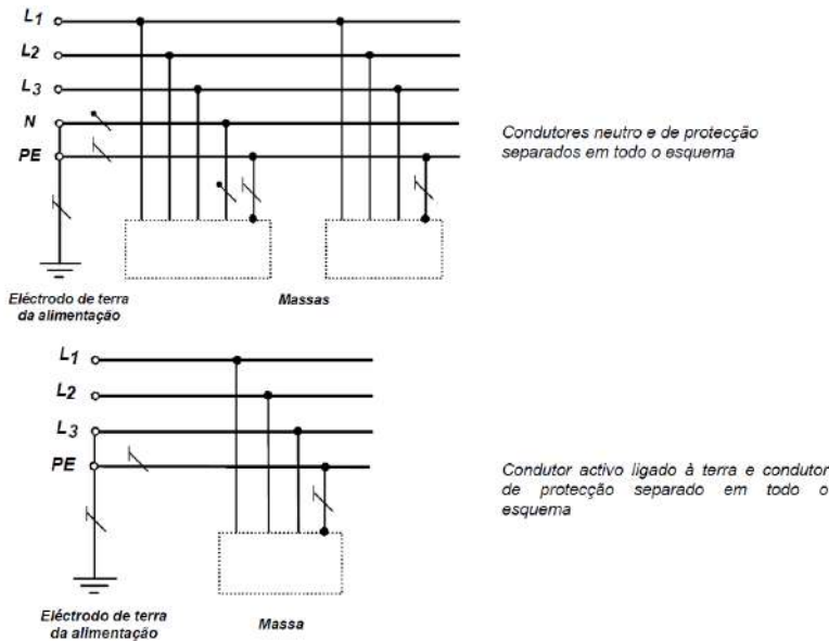
Fig. 31A — Esquema TN-S em corrente alternada (ac)
