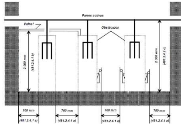
Fig. 48A — Passagem para serviço ou para manutenção nas instalações com proteção por meio de obstáculos
