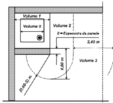
f) chuveiro sem bacia de receção e com parede fixa
