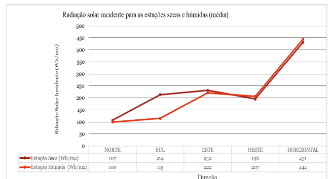
Gráfico 6: Média da Radiação Solar em Cabo Verde
