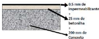
Figura 7 -Constituição dos Telhados em Cabo Verde
